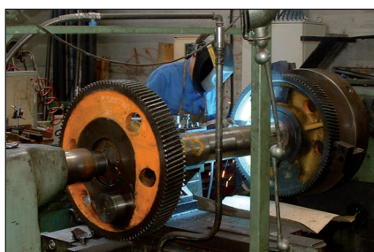
Train d'engrenage pour cartonnerie D 750 /2600
