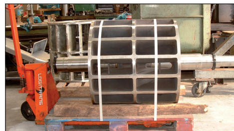
Gros rotor de pompe inox Diamètre 700/ 2250 mm.
